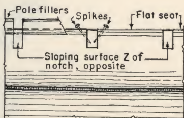
ELEVATION B
